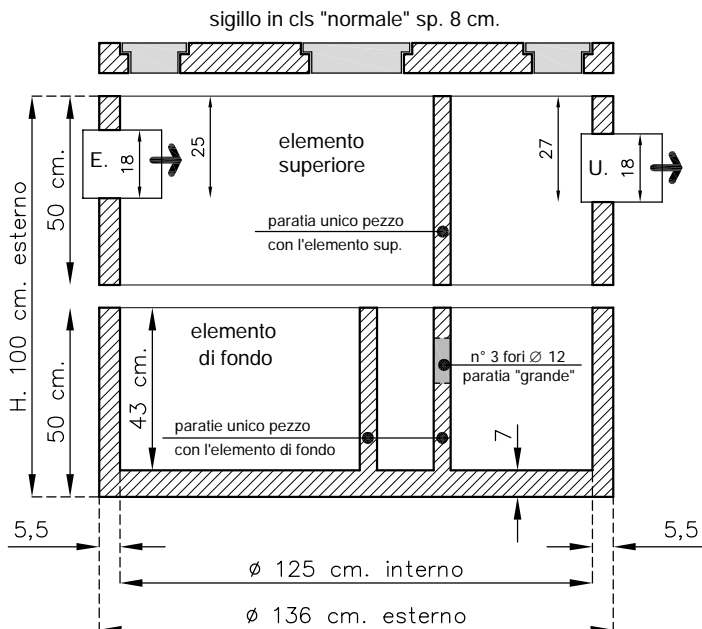
sezione A-A sc. 1:20
