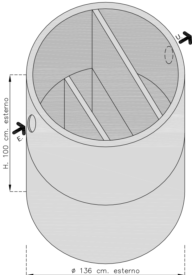
VASCA CONDENSAGRASSI DIAMETRO 125 NR. 2 ELEMENTI COMPRESO PARATIE
